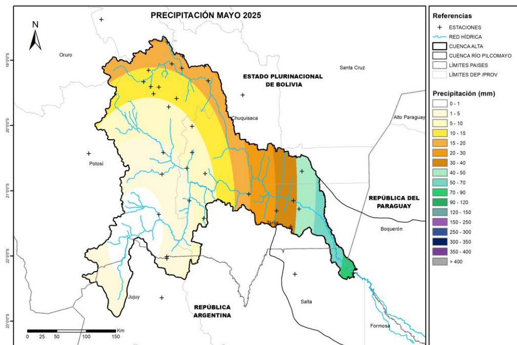
Imagen N°2: Lluvias en la Cuenca Alta del río Pilcomayo - Precipitación Acumulada May/2025
