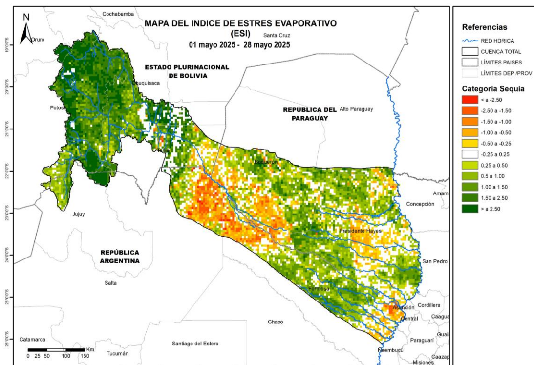
Imagen N°20: Mapa de Índice de Estrés Evaporativo (ESI) – Periodo: 01/05/2025 a 28/05/2025.
