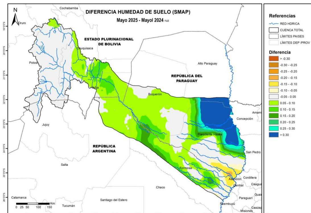
Imagen N°19: Diferencia de humedad de suelo - May/2025 - May/2024.
