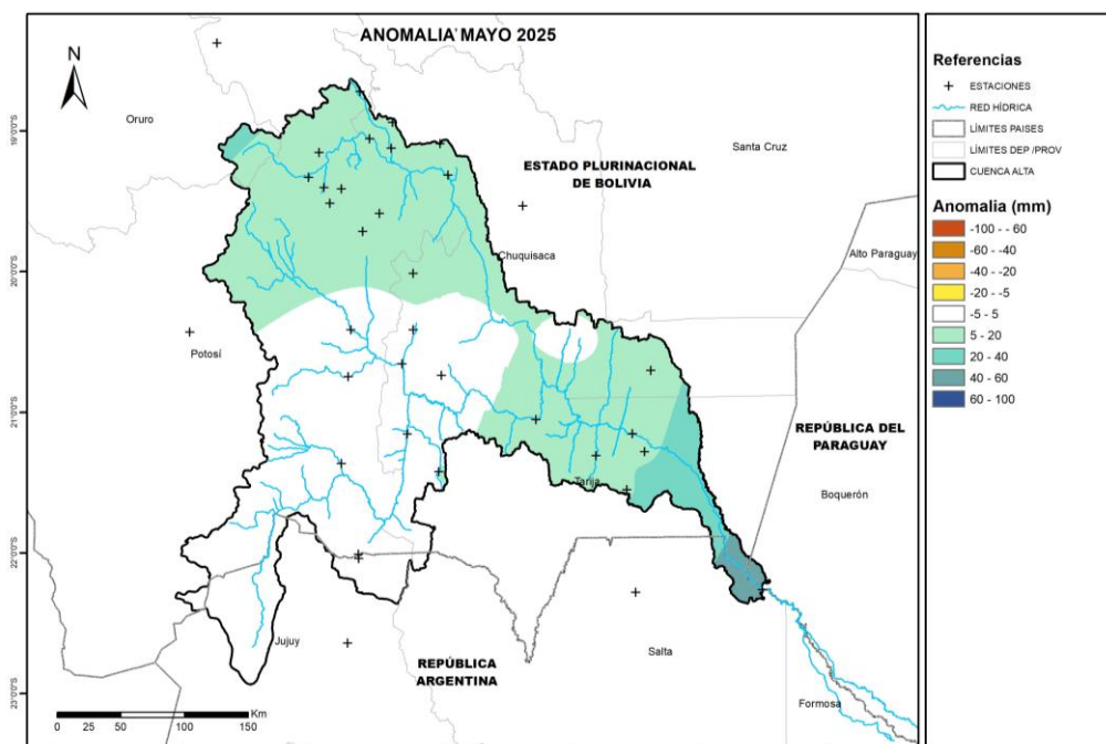
Imagen N°3: Anomalías lluvias - Mayo/2025
