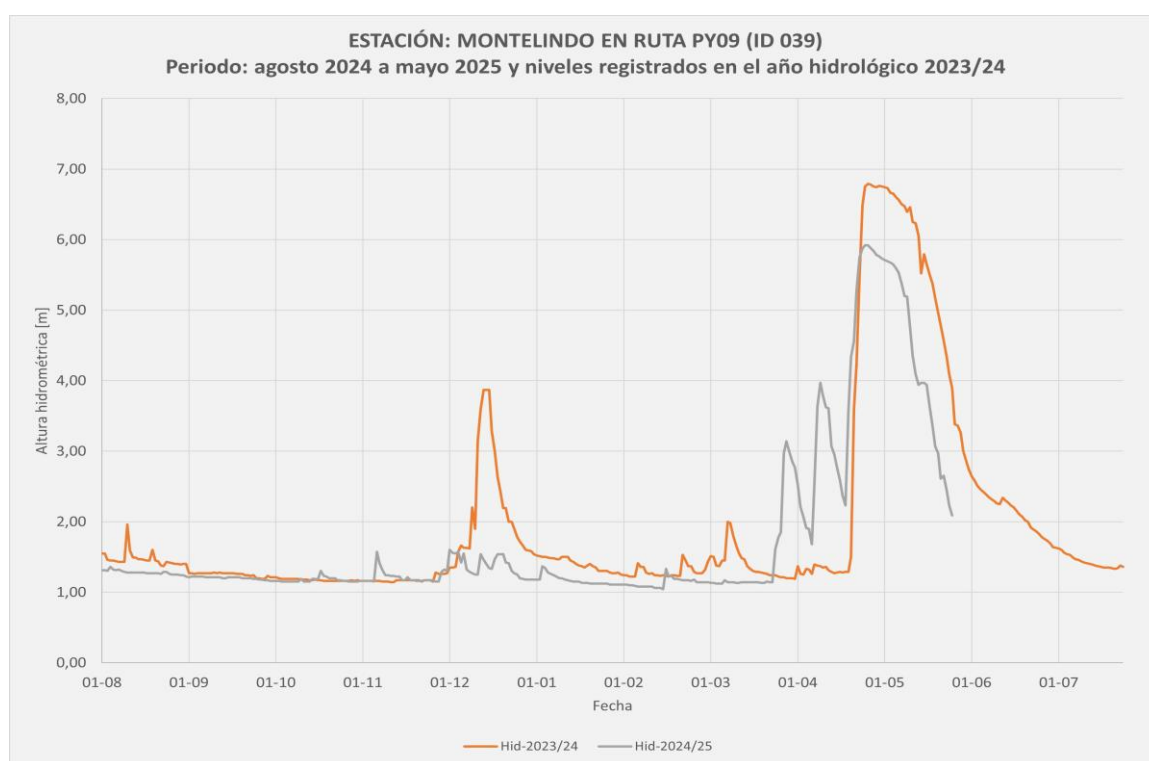
Imagen N°18: Evolución de los niveles hidrométricos - Estación Río Montelindo - RPY N°09 (ID 039)
